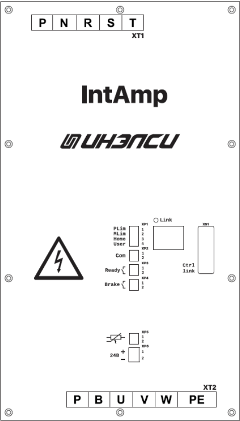
Рисунок 1 – Внешний сервоусилителей серии IntAmp-22/30/45
