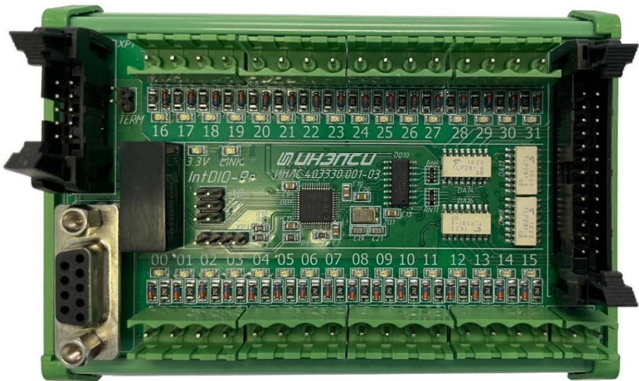
Рисунок 1 – Внешний вид модуля дискретных входов/выходов IntDIO-Pr
